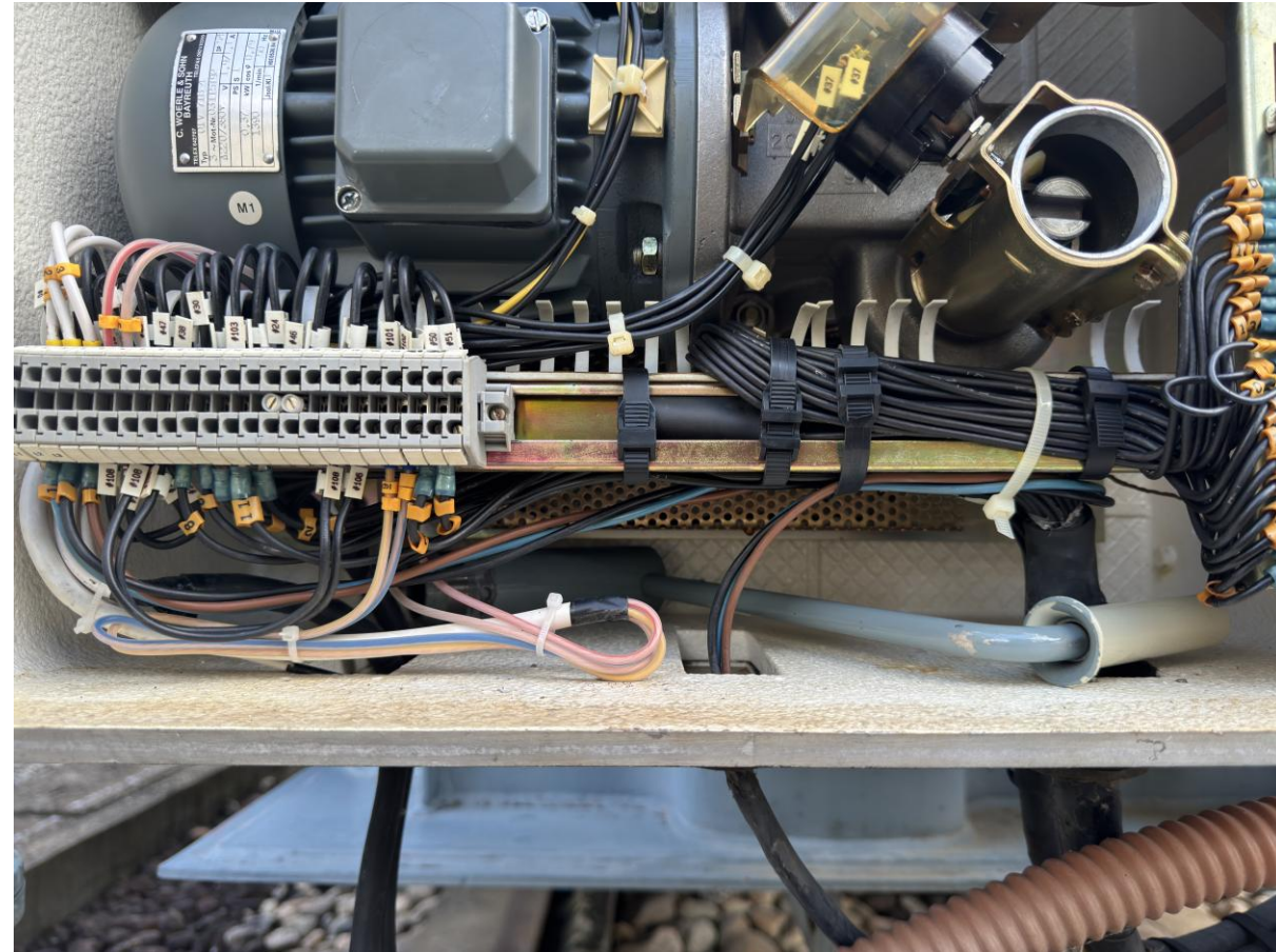
VIII.10 - Động cơ motor chuyển nấc phân áp
