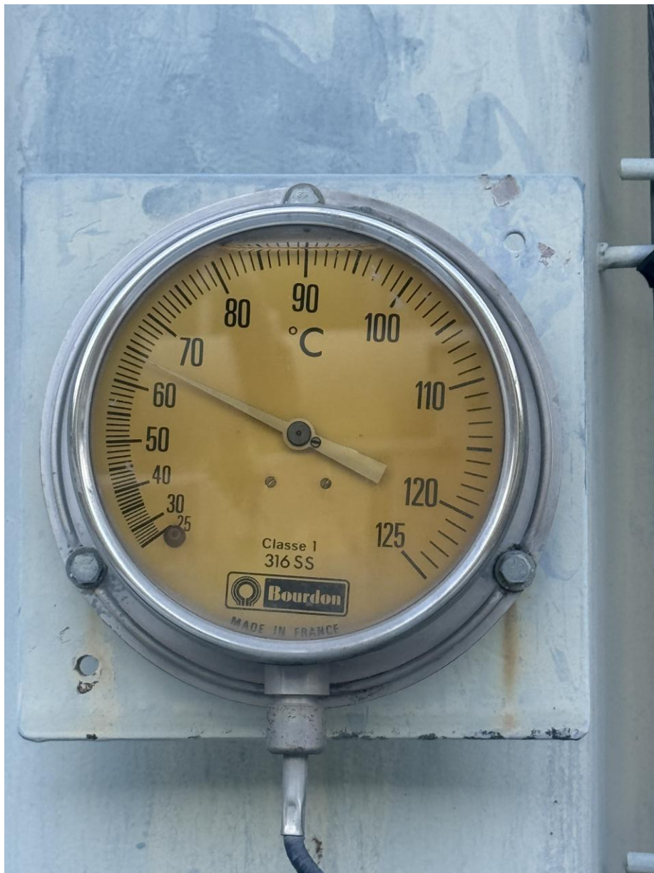
VIII.4 - Đồng hồ quan sát nhiệt độ dầu MBA chính
