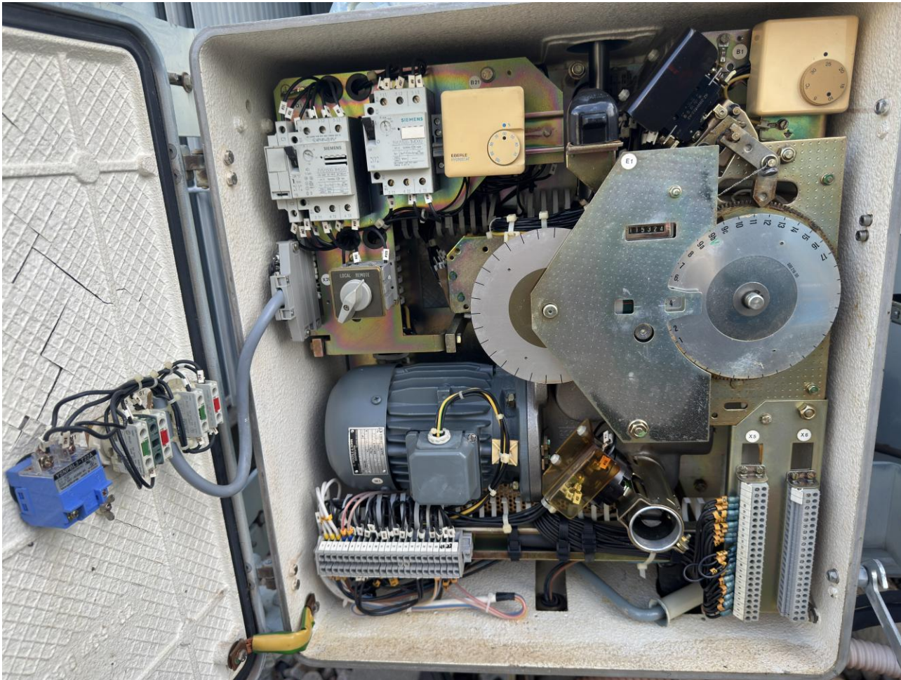
VIII.9 - Tủ nấc phân áp MBA
